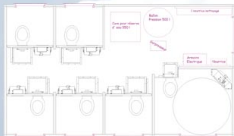
Bâtiment existant de 4 à 12 toilettes.
